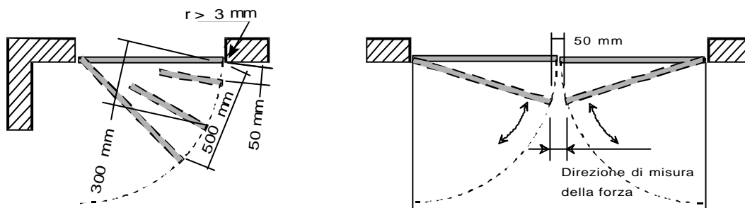
Figura 4: larghezze di apertura tra l'anta di una porta su cardini e il bordo opposto di chiusura
